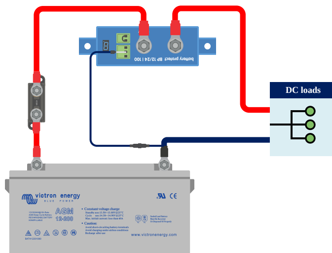
BatteryProtect en un sistema sencillo con puente entre los dos pines del conector terminal remoto (predeterminado de fábrica)
