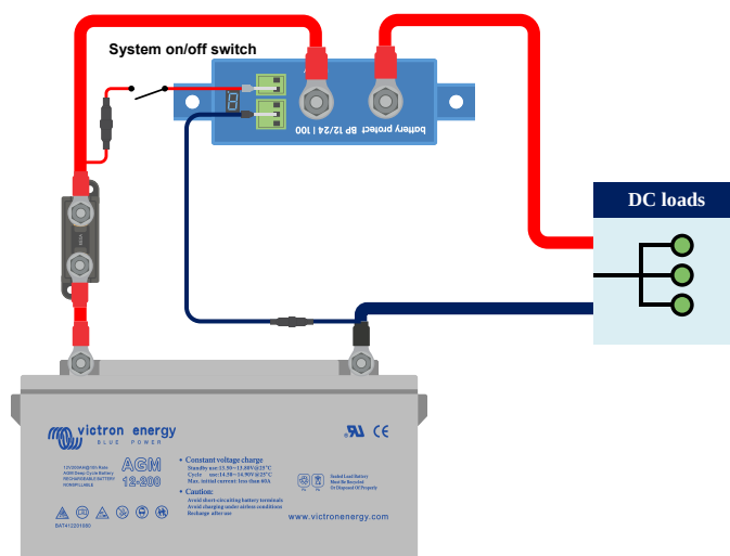
Interruptor conectado entre el positivo de la batería y el pin REMOTE del terminal remoto
