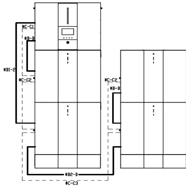
4 Módulos de Batería
